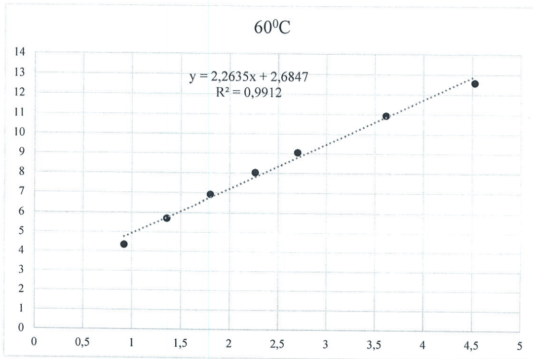
Зависимость удельной электропроводности рабочих растворов «Солжин» от концентрации при 60°C
