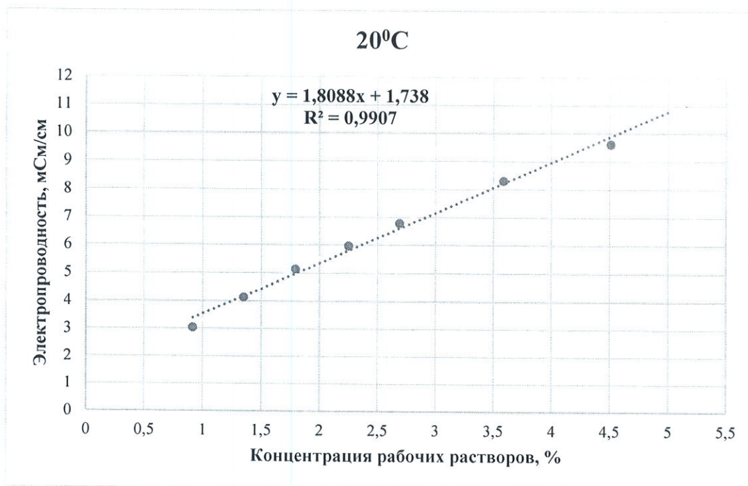
Зависимость удельной электропроводности рабочих растворов «Солжин» от концентрации при 20°C
