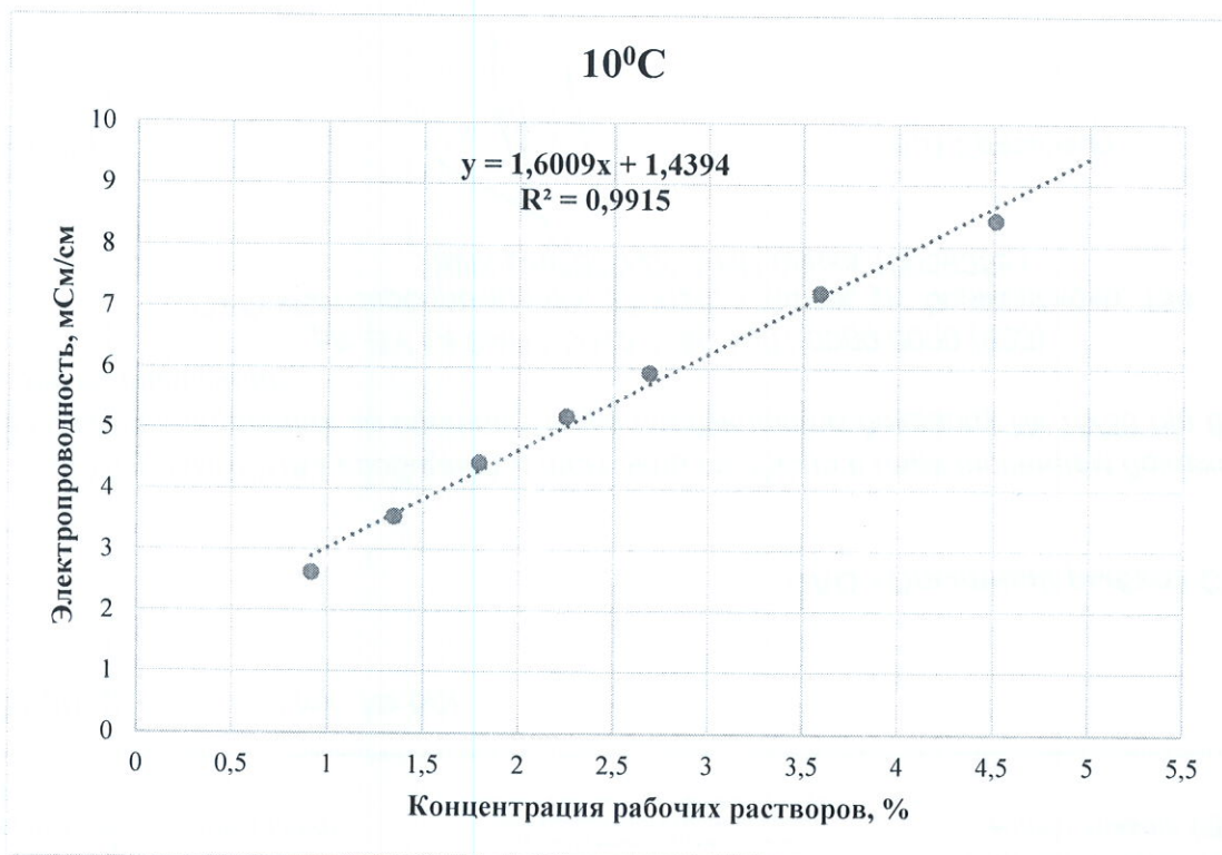
Зависимость удельной электропроводности рабочих растворов «Солжин» от концентрации при 10°C
