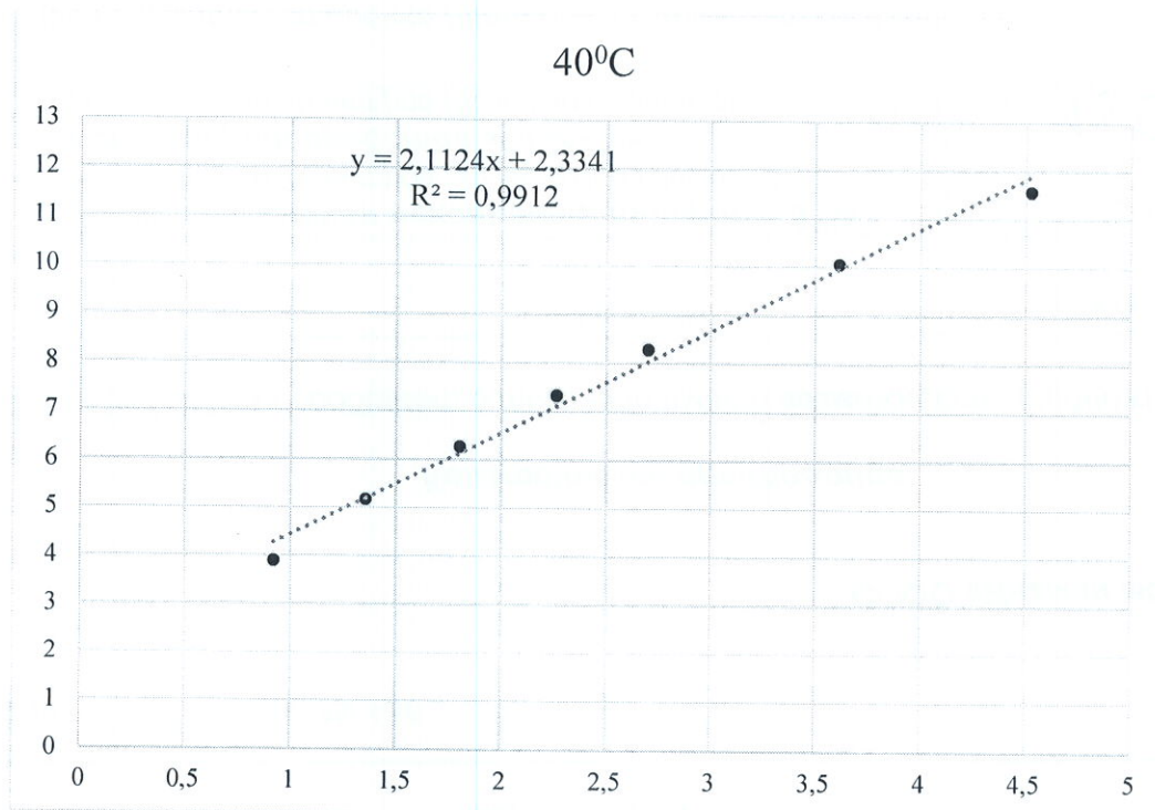
Зависимость удельной электропроводности рабочих растворов «Солжин» от концентрации при 40°C
